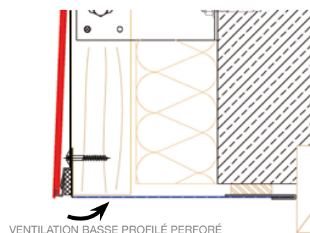
DÉTAIL LINTEAU
