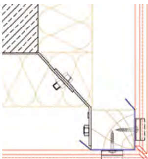
ANGLE SORTANT SANS PROFILÉ
