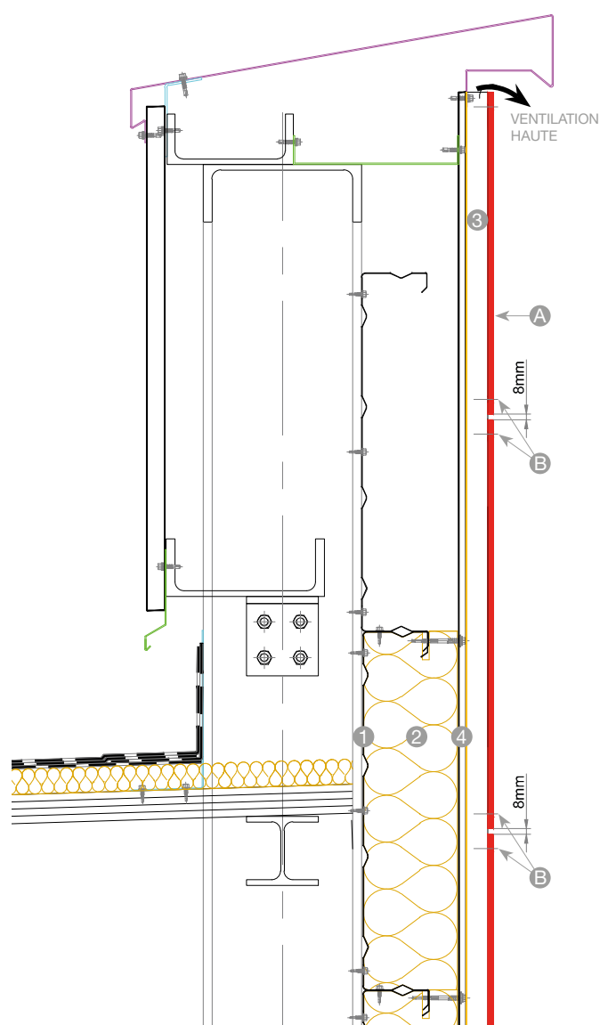
DÉTAILS POINT HAUT
