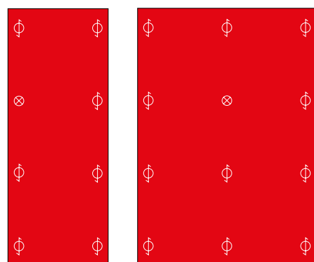
POSE SUR 2 APPUIS
