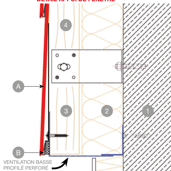
DÉTAIL DÉPART BAS
