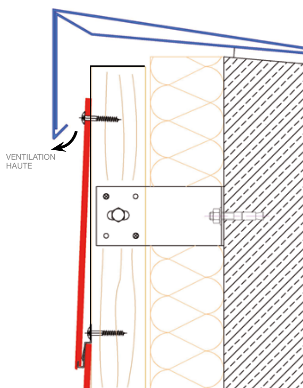
DÉTAIL COUVERTINE
