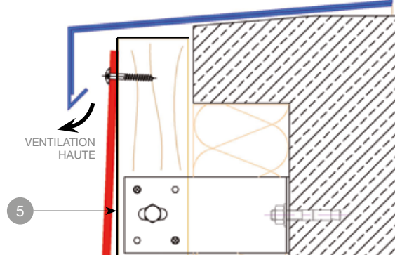
DÉTAIL APPUI DE FENÊTRE
