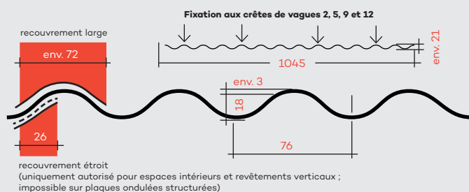
Coupe transversale du PLEXIGLAS® Resist WP 76/18/3
