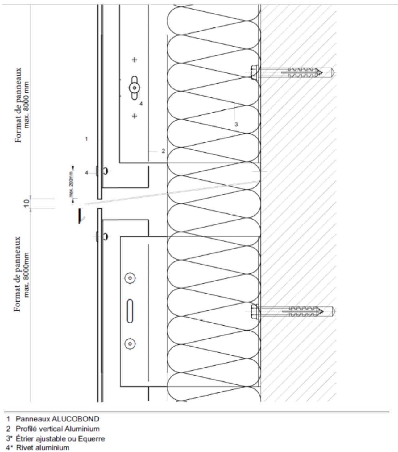
Figure 17b – Jonction de dilatation profil vertical – Coupe verticale Système riveté / vissé
