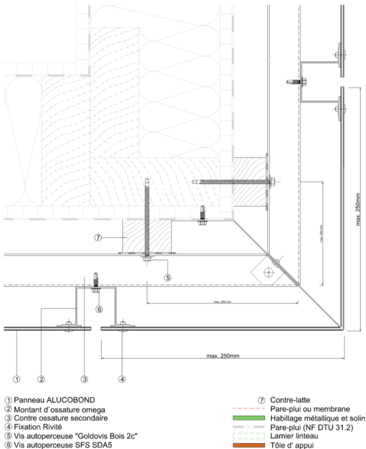
Figure 25 – Pose sur COB – Coupe verticale - Triple réseau - Système riveté / vissé - Angle rentrant
